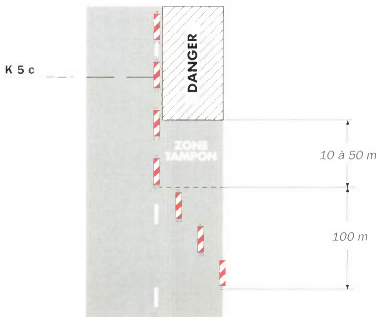
Schéma n°2
